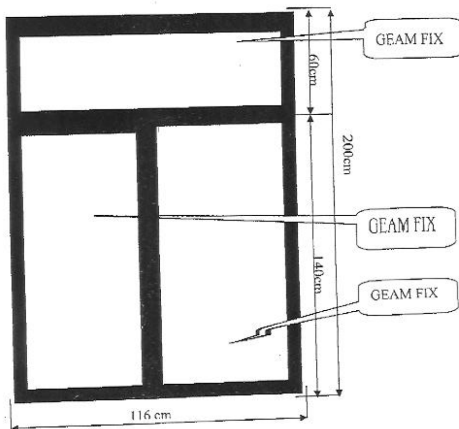
SCHIȚĂ GEAM 2
