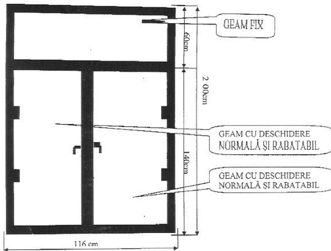
SCHIȚĂ GEAM 1
